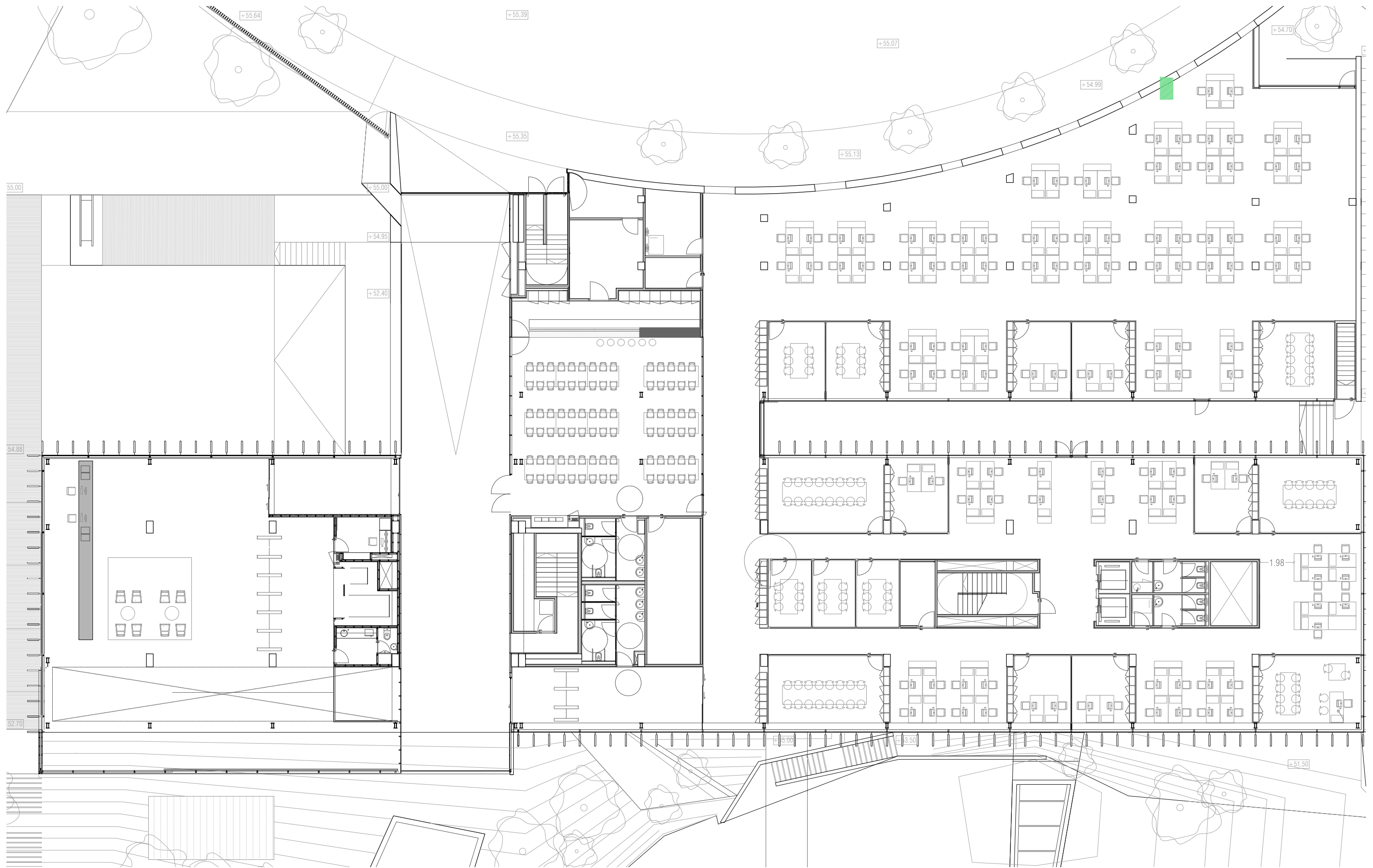
PLANTA BAIXA
